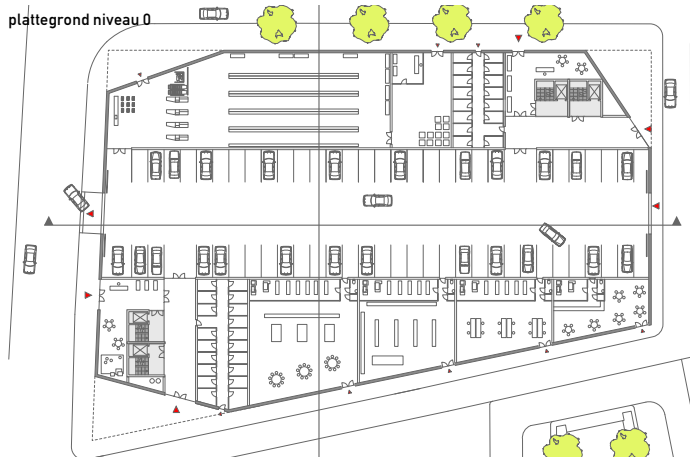
plattegrond niveau 0
