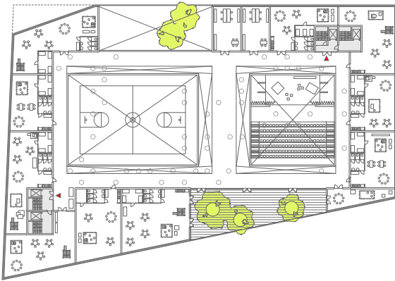
plattegrond niveau +2
