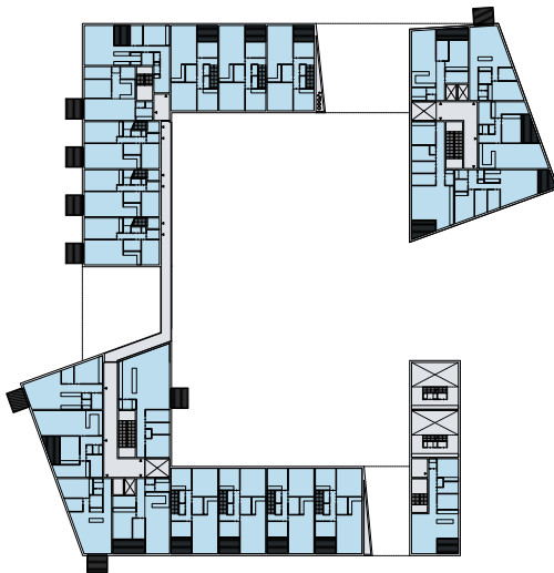
plattegrond niveau 0
